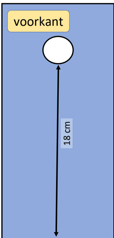
onderdelen en afmetingen voor nestkast (koolmees, pimpelmees)
